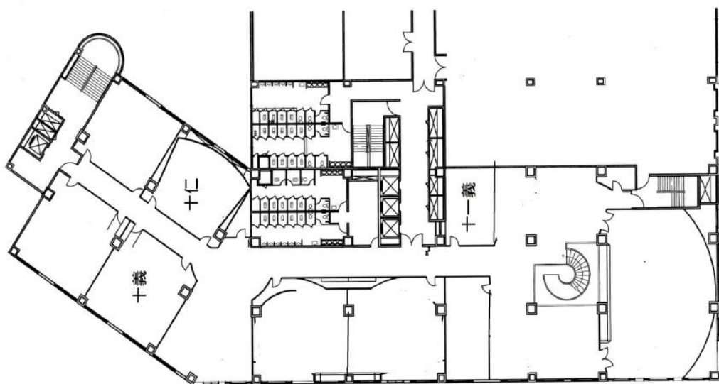
光復中學綜合大樓東側三樓教室配置圖
